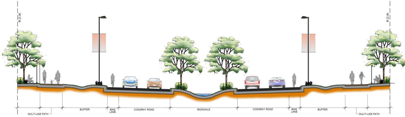
ຕົວຢ່າງຮູບຕັດທາງ ປະເພດທີ 1 例子道路剖面图第一种
