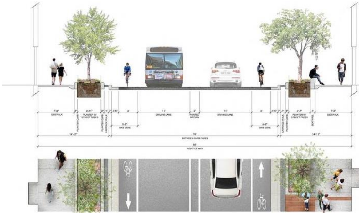
ຕົວຢ່າງຮູບຕັດທາງ ປະເພດທີ 2 例子道路剖面图第二种
